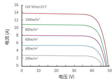
电流-电压曲线 (LR5-72HBD 530M)
