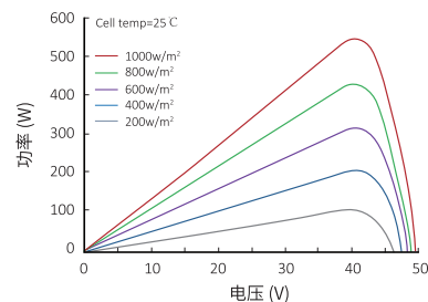
功率-电压曲线 (LR5-72HBD 530M)
