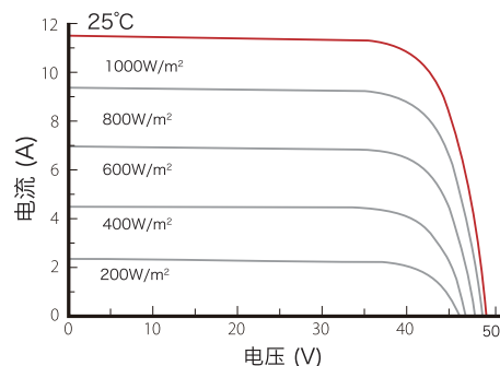
电流-电压曲线 (LR4-72HBD 445M)
