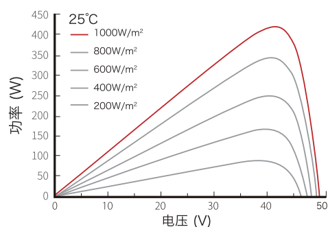
功率-电压曲线 (LR4-72HBD 445M)
