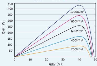
组件的P-V曲线(440W)
