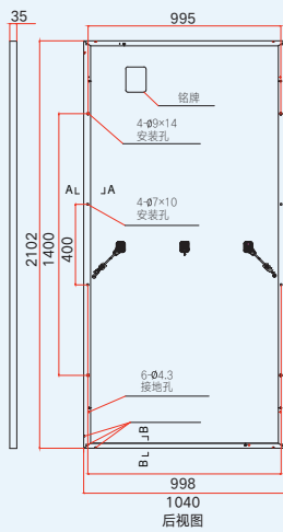
后视图
